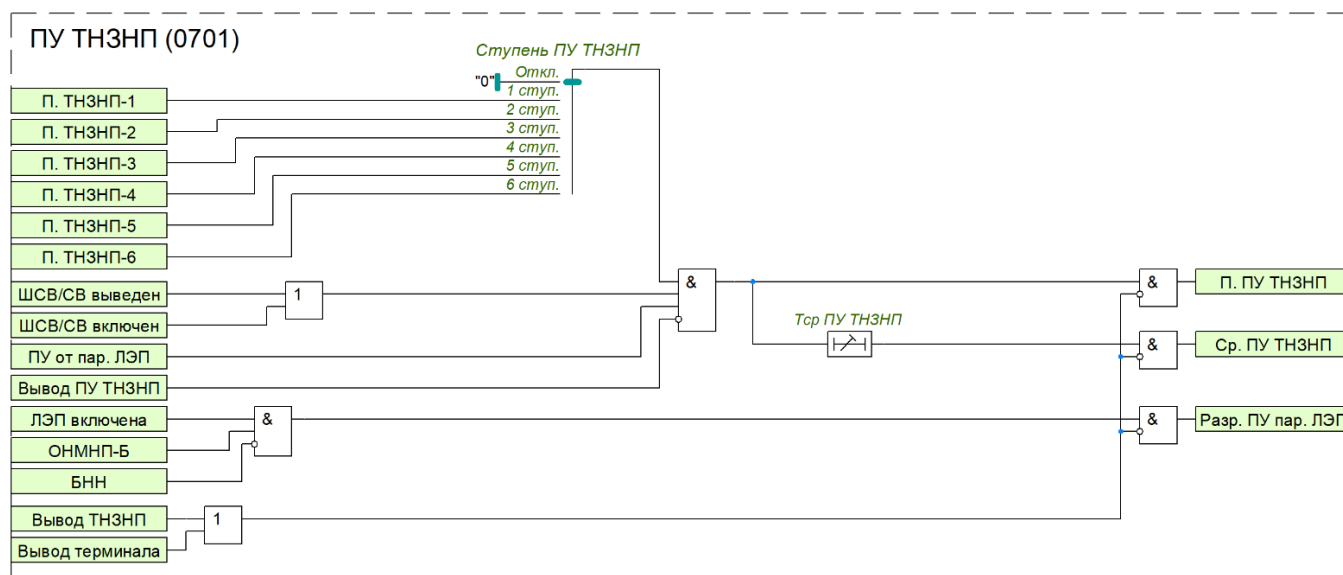
Рисунок 1.24 – Функциональная схема пуска ПУ TH3NP
